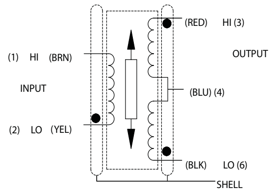
WIRING SCHEMATIC
