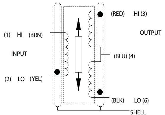
WIRING SCHEMATIC
