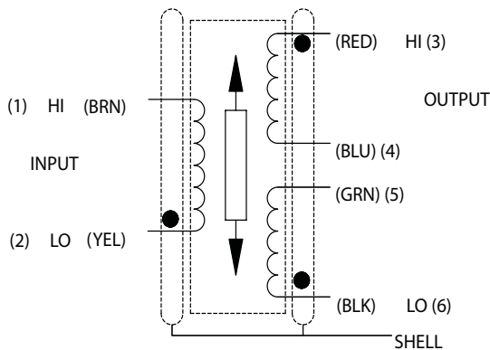
WIRING SCHEMATIC
