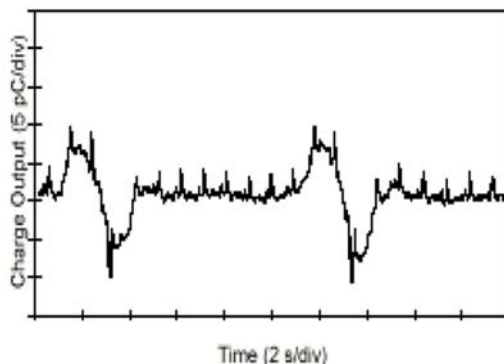
图2 放在垫子和铺有地毯的地面之间时的响应
