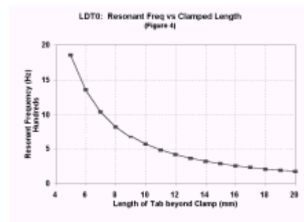
图 4: 谐振频率与
